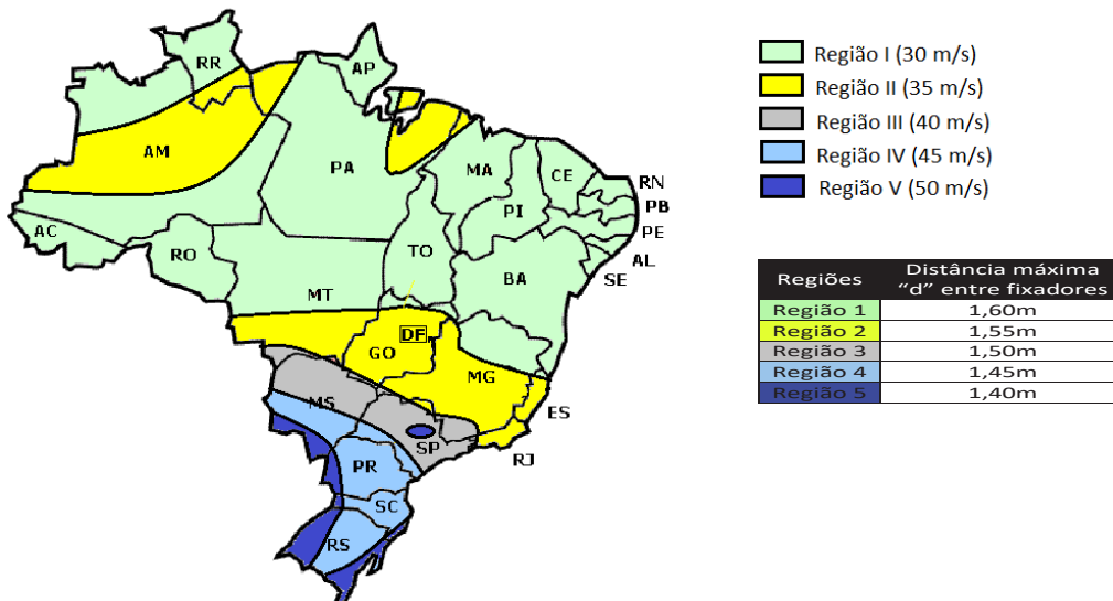
Gráfico das isopleias de velocidade básica dos ventos (NBR-6123)
